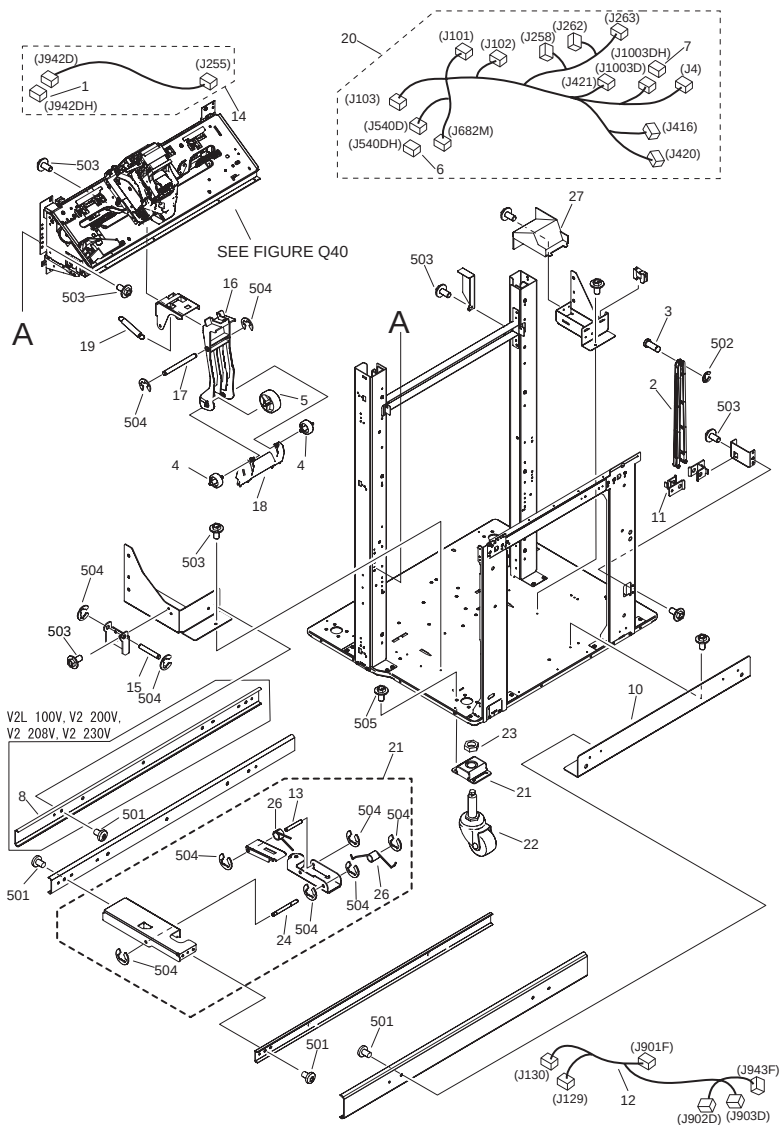
FIGURE Q13 INTERNAL COMPONENTS 3
